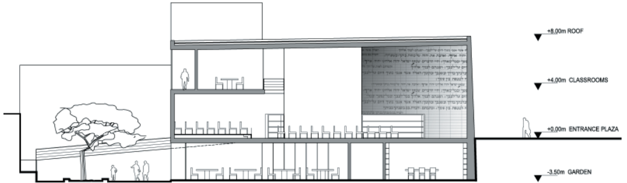
LONGITUDINAL SECTION
